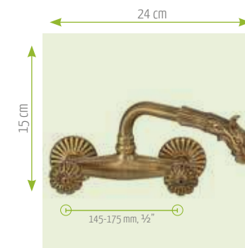
Art. 1150 (Anschl./Collegam./Conn. ½") Warm-/Kaltwassermischer Mescolatore acqua calda/fredda Warm/cold water mixer
