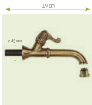
Art. 1200 (Anschl./Collegam./Conn. ½") Wasserhahn mit Schlauchanschluss Rubinetto con presa tubolare Water tap with hydraulic hose
