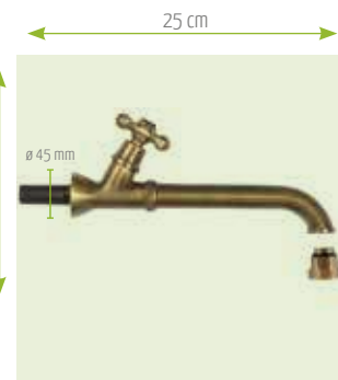
Art. 1230 (Anschl./Collegam./Conn. ½") Wasserhahn mit Schlauchanschluss Rubinetto con presa tubolare Water tap with hydraulic hose
