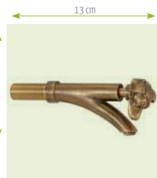
Art. 1100 (Anschl./Collegam./Conn. ½") Wasserhahn mit Druckknopf Rubinetto con pulsante Water tap with pushbutton
